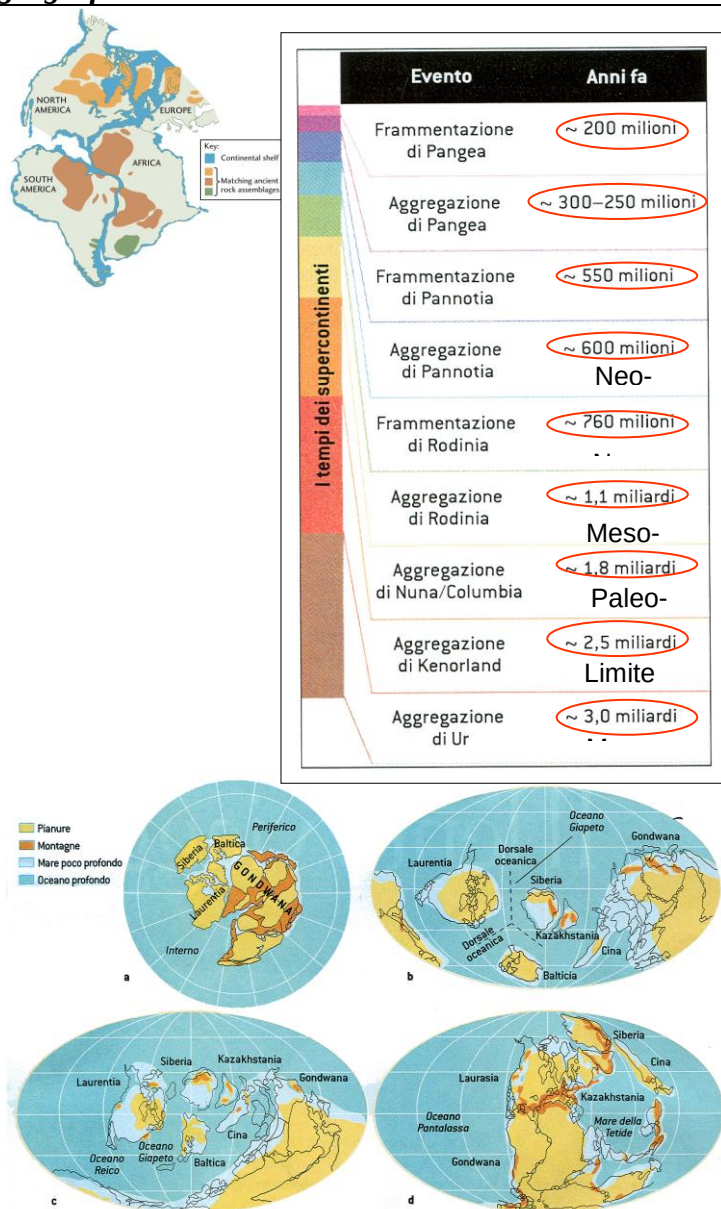
I grandi supercontinenti nella storia della terra
