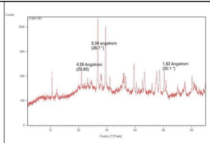
Fig. 3. Il diffrattogramma X del quarzo. Ogni picco corrisponde ad una precisa famiglia di piani reticolari propria del minerale stesso.
